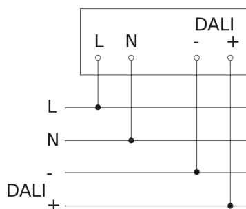
Diagrama electrónico maestro
